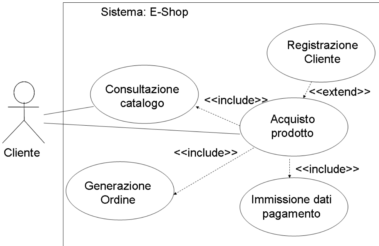
Fig. 4.6: esempio di casi d'uso di un sistema E-Shop collegati fra loro da relazioni di include ed extend.
