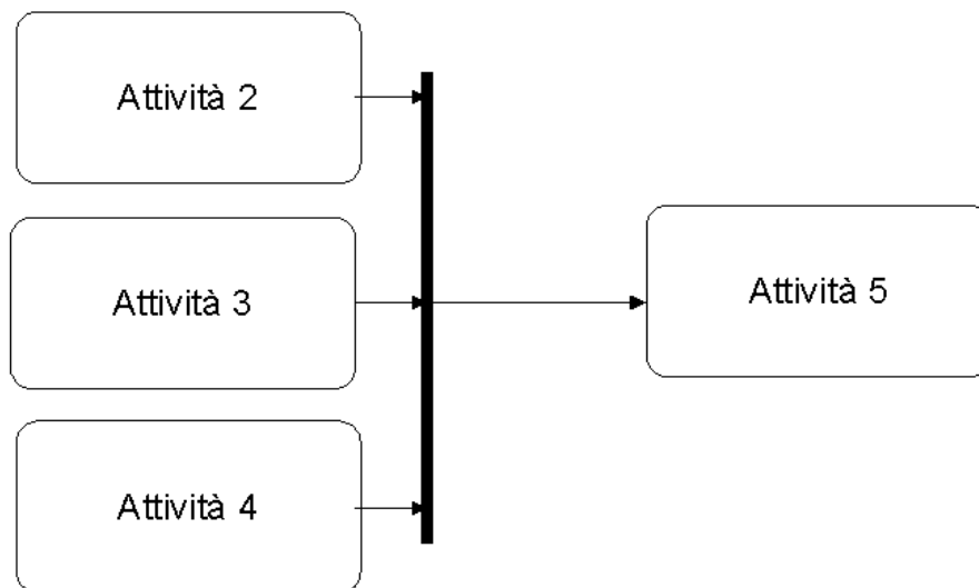
Fig. 4.9: And-split.
